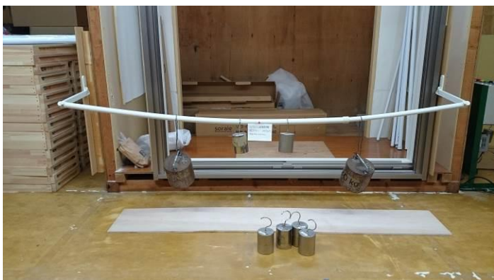
48kgf 負荷
